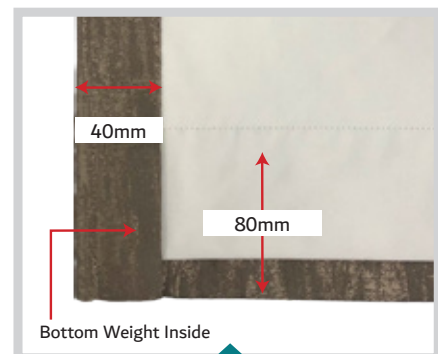
Side & Bottom Hem
